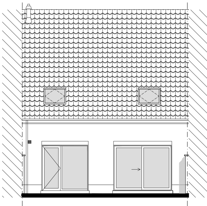
Achtergevel
