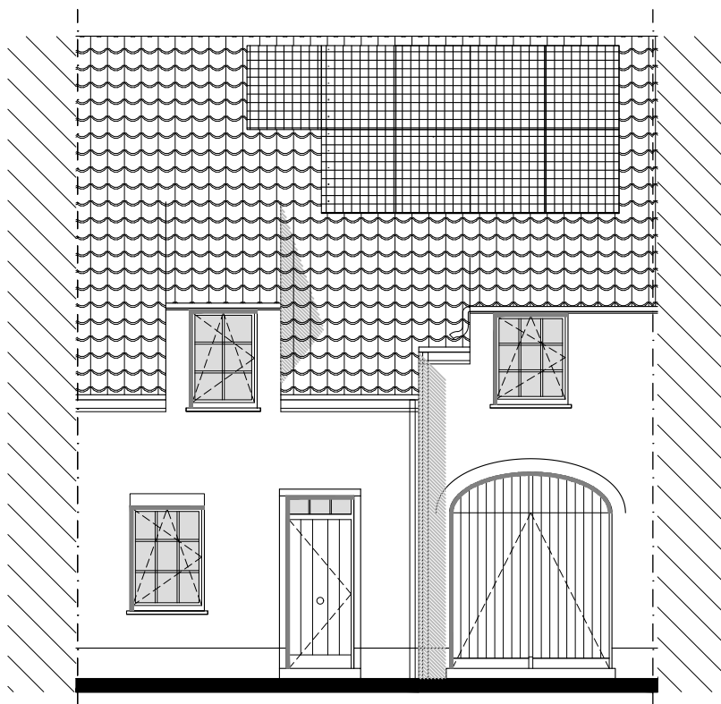
Voorgevel
