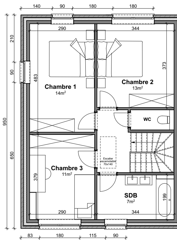
Plan étage
