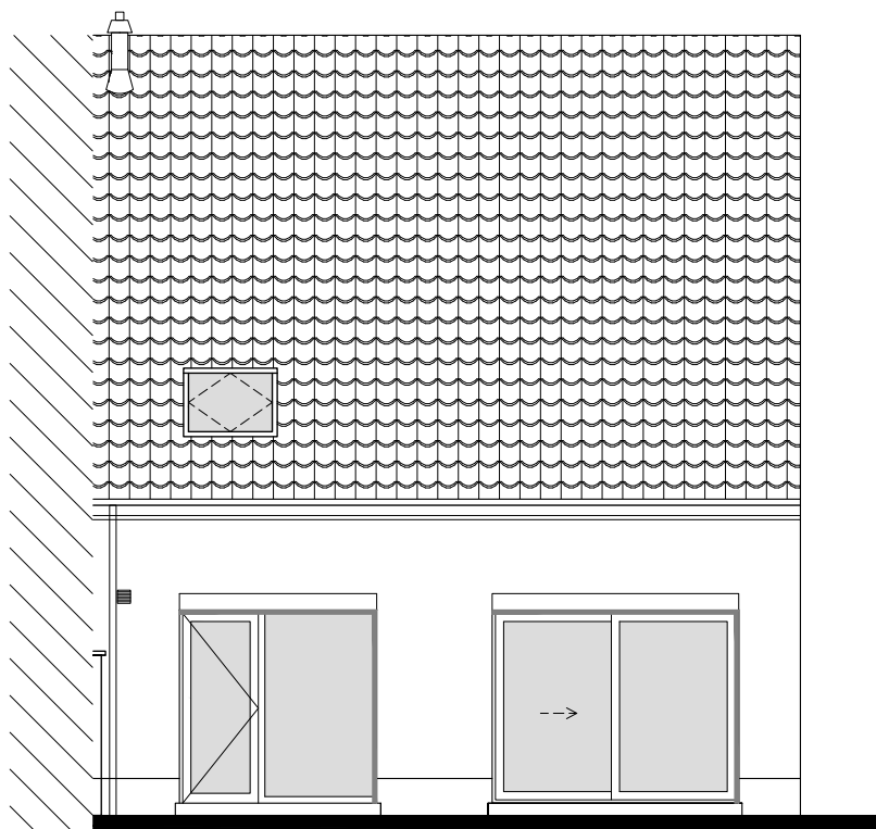
Achtergevel
