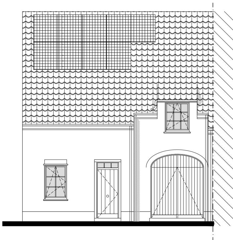
Vorgevel
