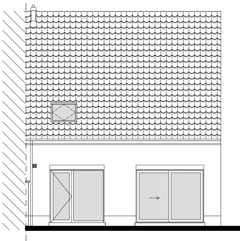
Achtergevel
