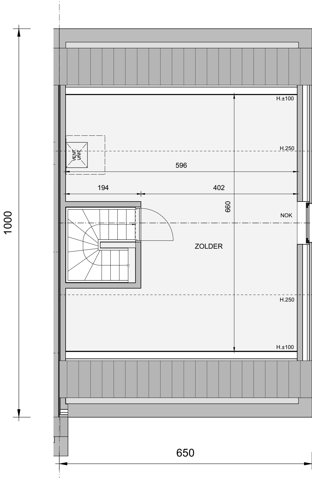
Zolder (optioneel af te werken)
