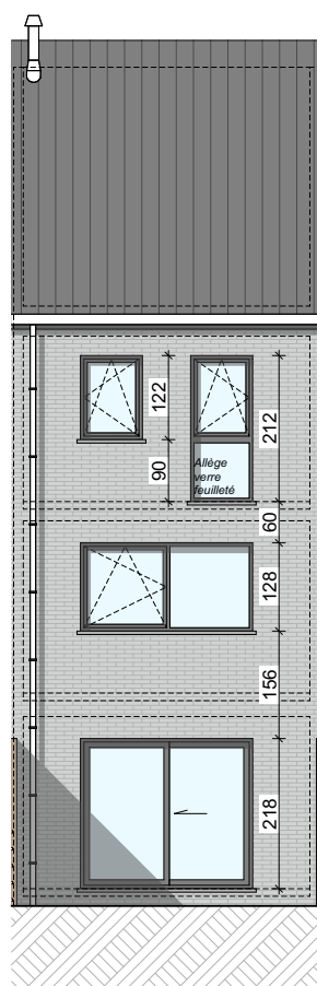
Façade arrière
