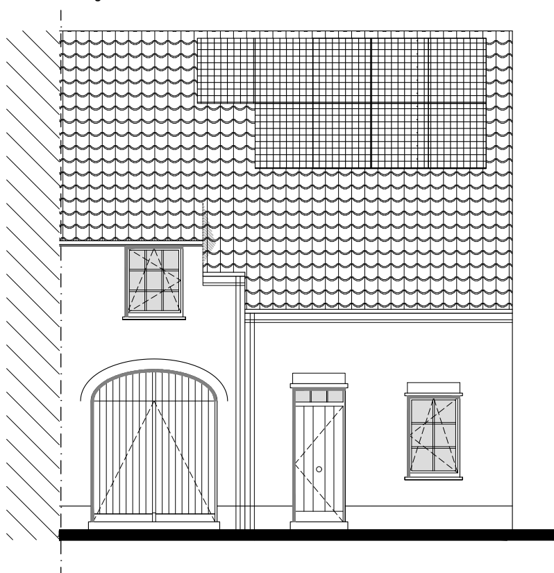
Voorgevel
