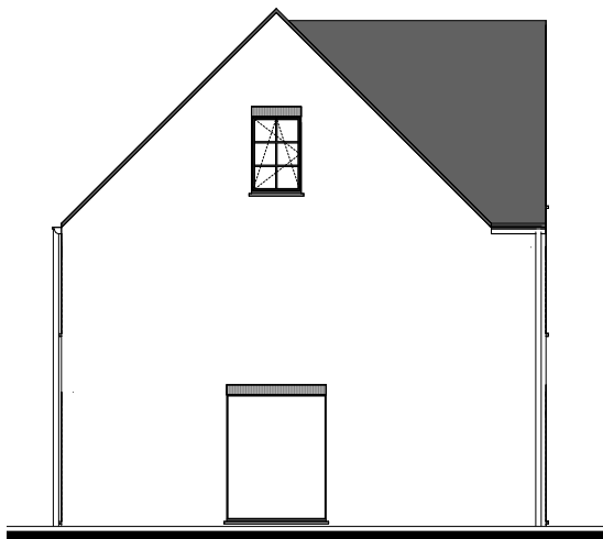
Zijgevel links
