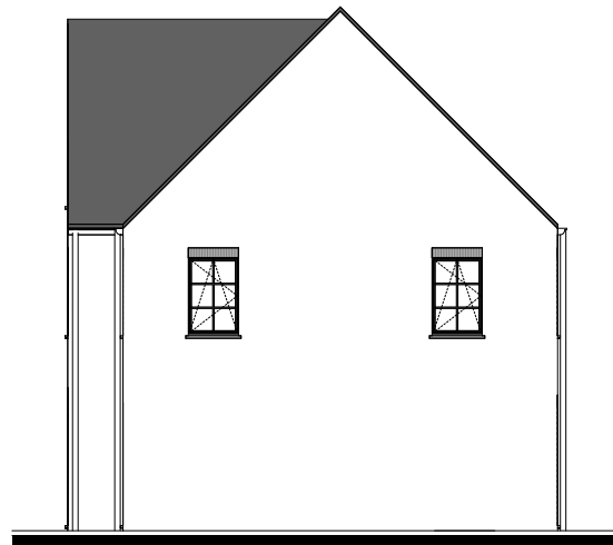
Zijgevel rechts
