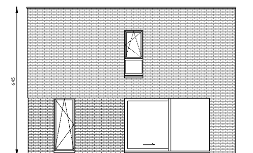
Tuingevel
