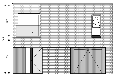
Voorgevel
