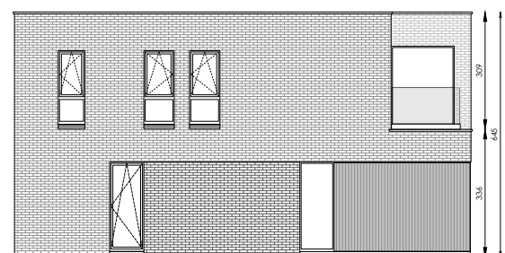
Zijgevel links
