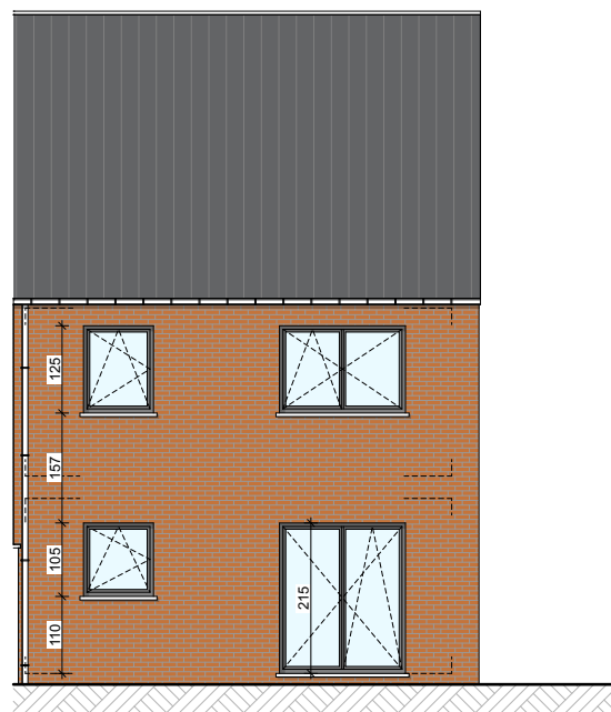
Façade arrière
