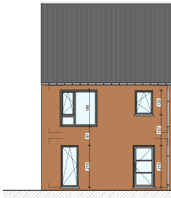
Façade avant
