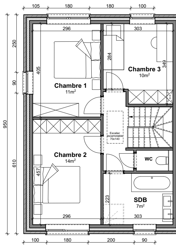
Plan étage
