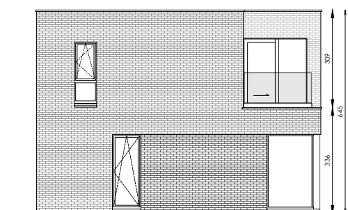
Zijgevel links
