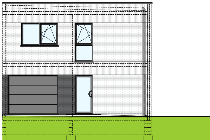
Façade avant
