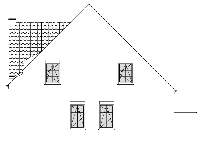
Zijgevel rechts
