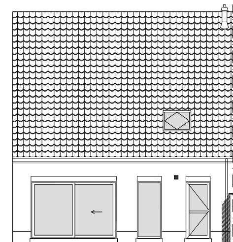
Achtergevel
