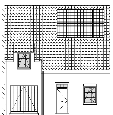
Voorgevel
