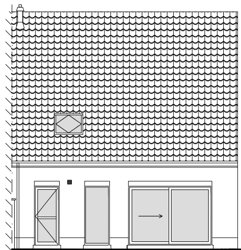
Achtergevel
