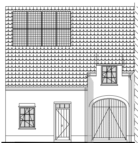
Voorgevel
