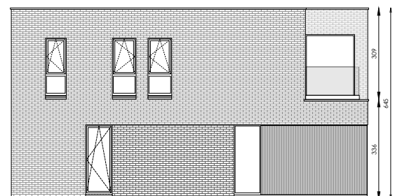
Zijgevel links
