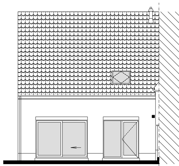
Achtergevel
