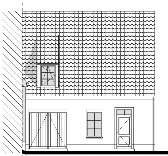
Voorgevel
