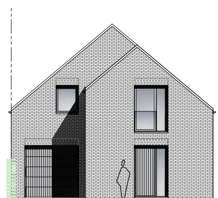
Vorgevel
