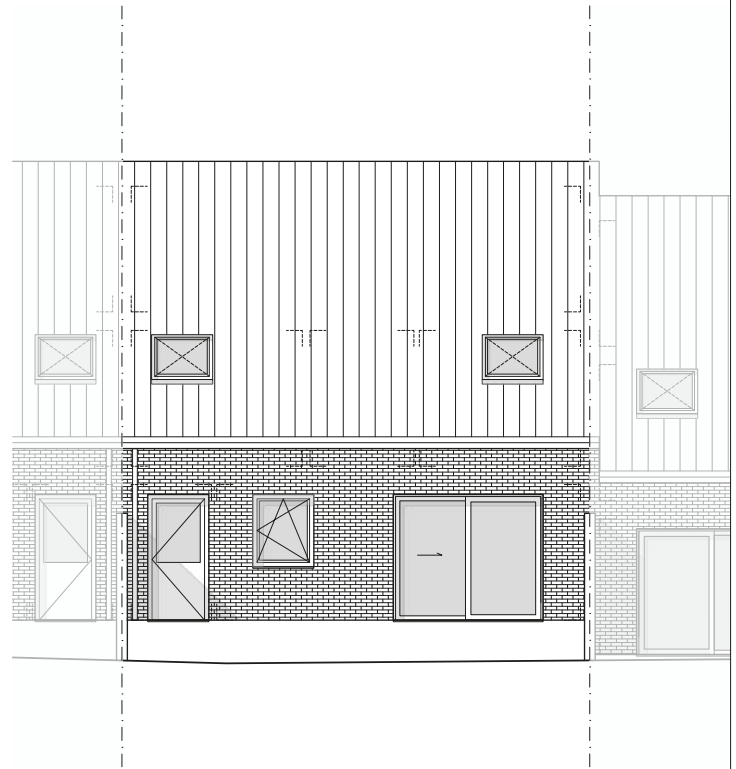
Achtergevel
