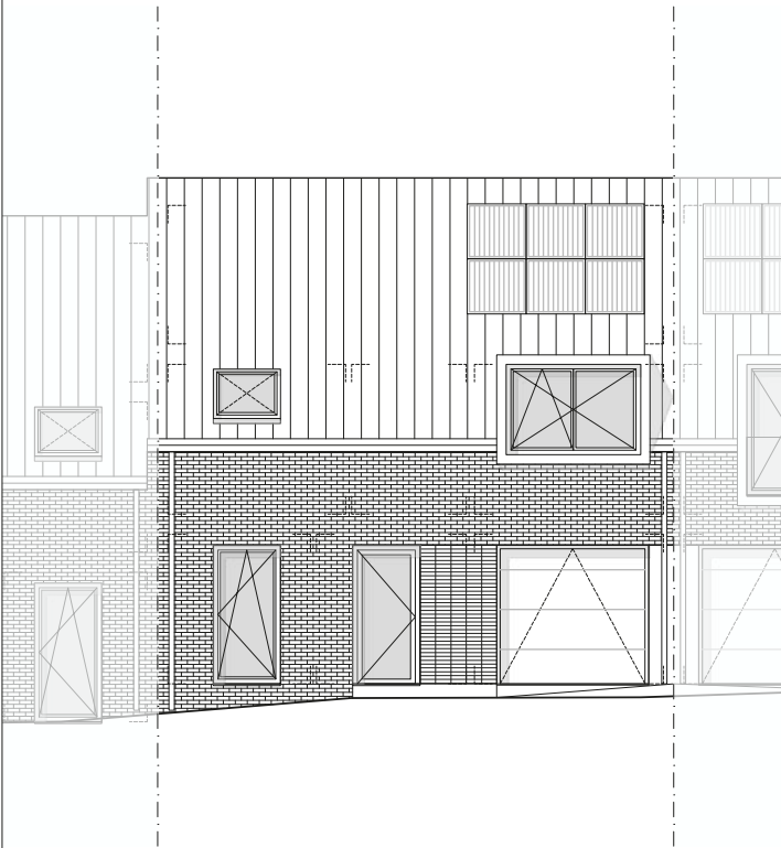
Voorgevel
